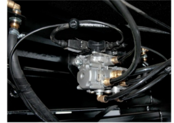
Рабочая тормозная система - WABCO , пневматическая, двухконтурный привод отдельно к тормозам передних и задних колес, тормозные механизмы барабанного типа на всех колесах, ABS .
